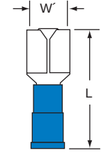
72F-250-32-NB Wire Range 16-14
