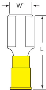
73F-375-50-NB Wire Range 12-10
