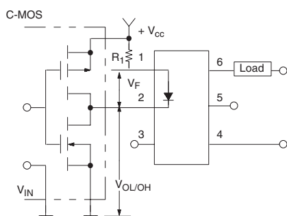
C-MOS
