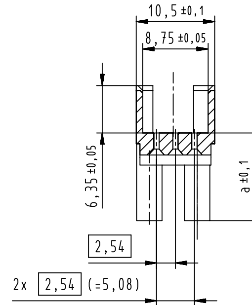
A-A (2:1)
