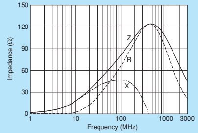
BLM15PX800SN1
