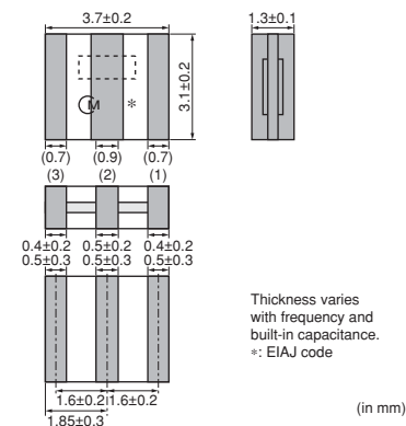
CSTCV_X_Q 20.01-70.00MHz
