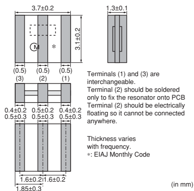
CSACV_X_Q 20.01-70.00MHz
