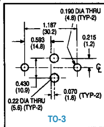
TO-3
