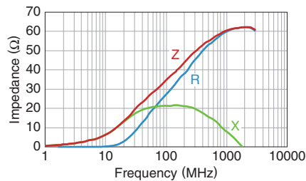
MPZ0603S330CT000
