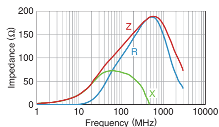
MPZ1005S121CT000
