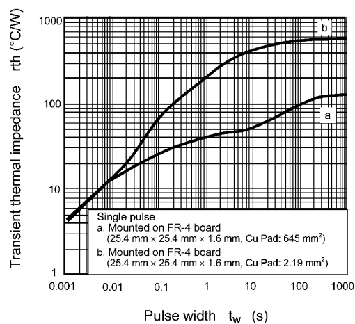
Fig. 7.13 r_{th} - t_w
