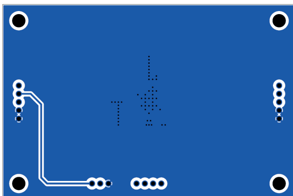
Layer 3 (GND)
