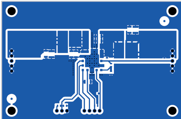
Top Layer
