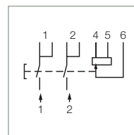
2602.5101
