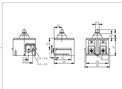
1246.3201 DPNO
