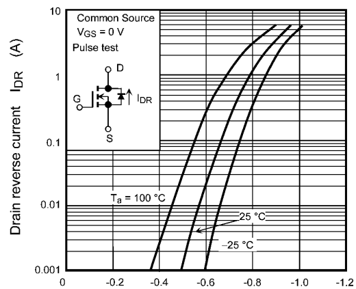
Fig. 7.8 I_{DR} - V_{DS}
