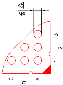
DETAIL : B
