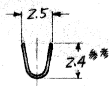
断面 A-A
