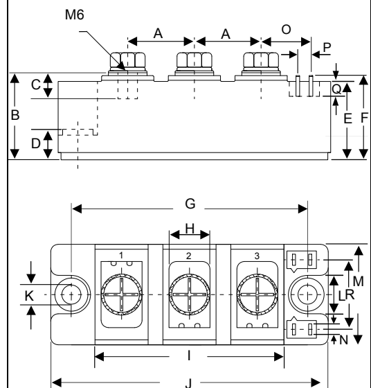
DIMENSIONS
