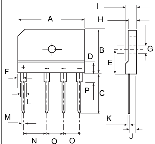
DIMENSIONS
