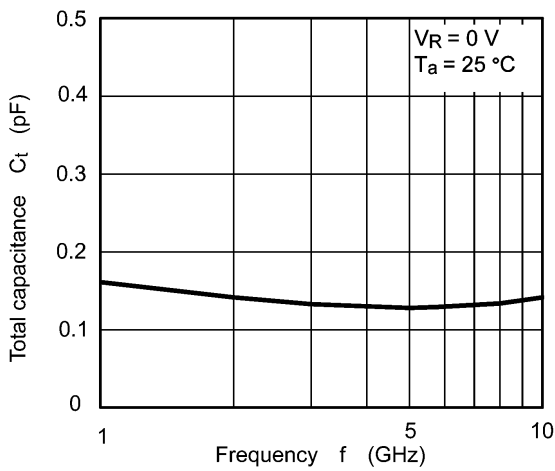
Fig. 9.4 C_t - f
