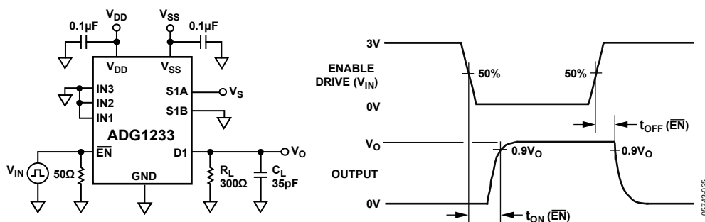
Figure 29. Enable Delay, t ON (EN), t OFF (EN)
