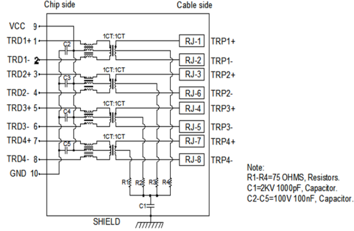
805 (2.5G Base-T)
