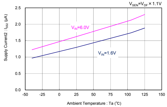
XC6134
