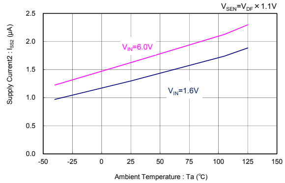
XC6134
