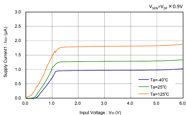
XC6134
