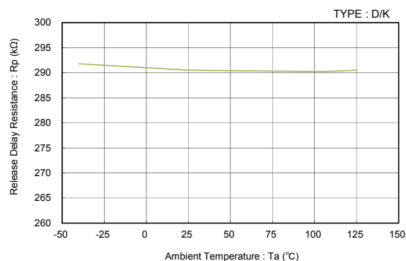
XC6134
