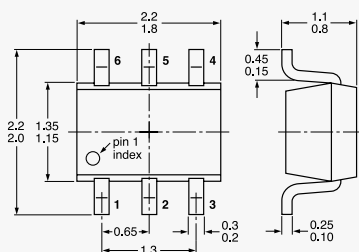
SOT363 (SC-88)
