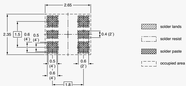
SOT363 (SC-88)
