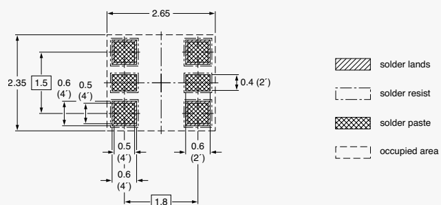
SOT363 (SC-88)
