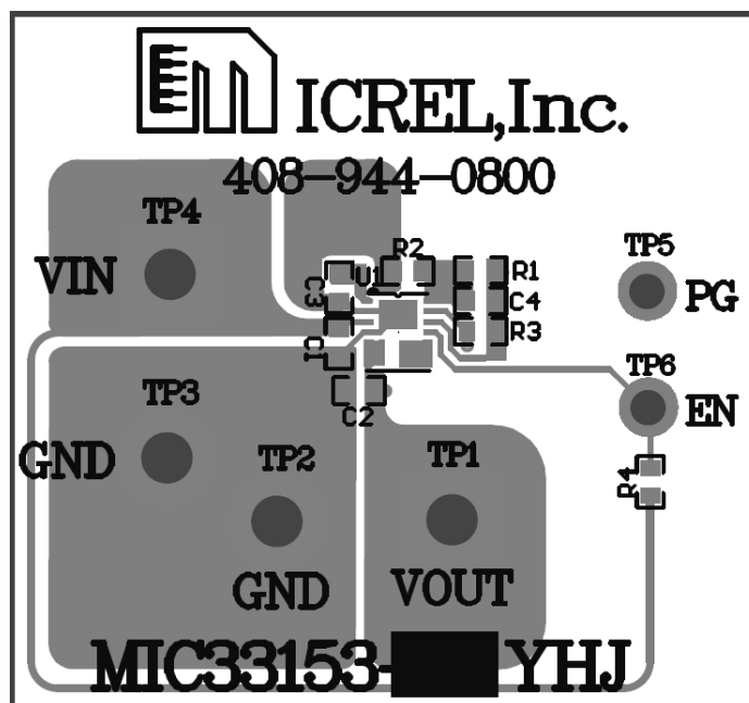
Top Layer
