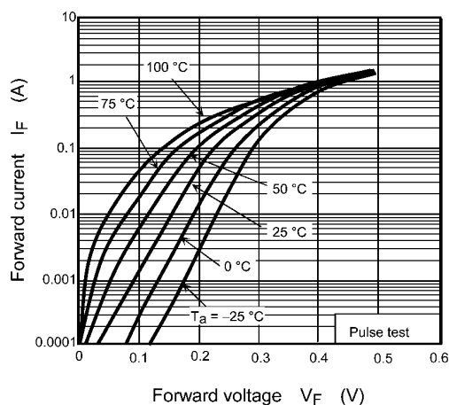
Fig. 9.1 I_F - V_F
