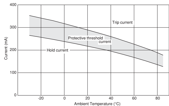
PTGL04AS100K2B51B0
