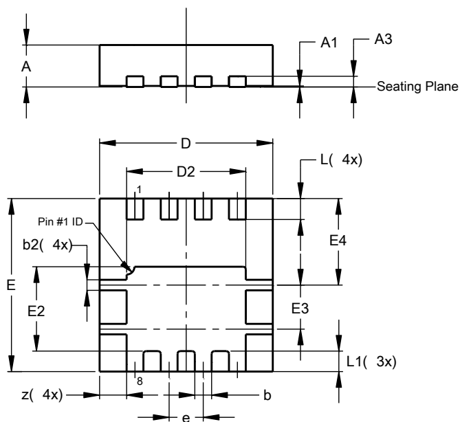
PowerDI3333-8
