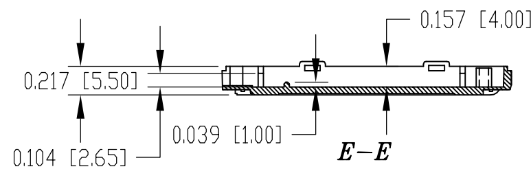
LID
