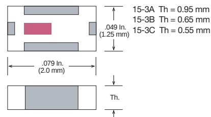
Case 15-3 (EIA 0805 / 2012)
