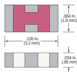
Case 18-2 (EIA 1206 / 3216)
