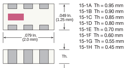
Case 15-1 (EIA 0805 / 2012)
