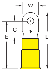
13-4S-NB Stud Size 4 Wire Range 12-10
