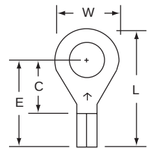
12-14S Stud Size 1/4 Wire Range 16-14
