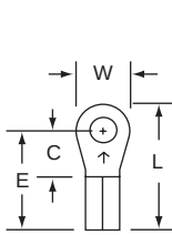
12-4S Stud Size 4 Wire Range 16-14
