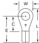
L-12-10 Stud Size 10 Wire Range 16-14
