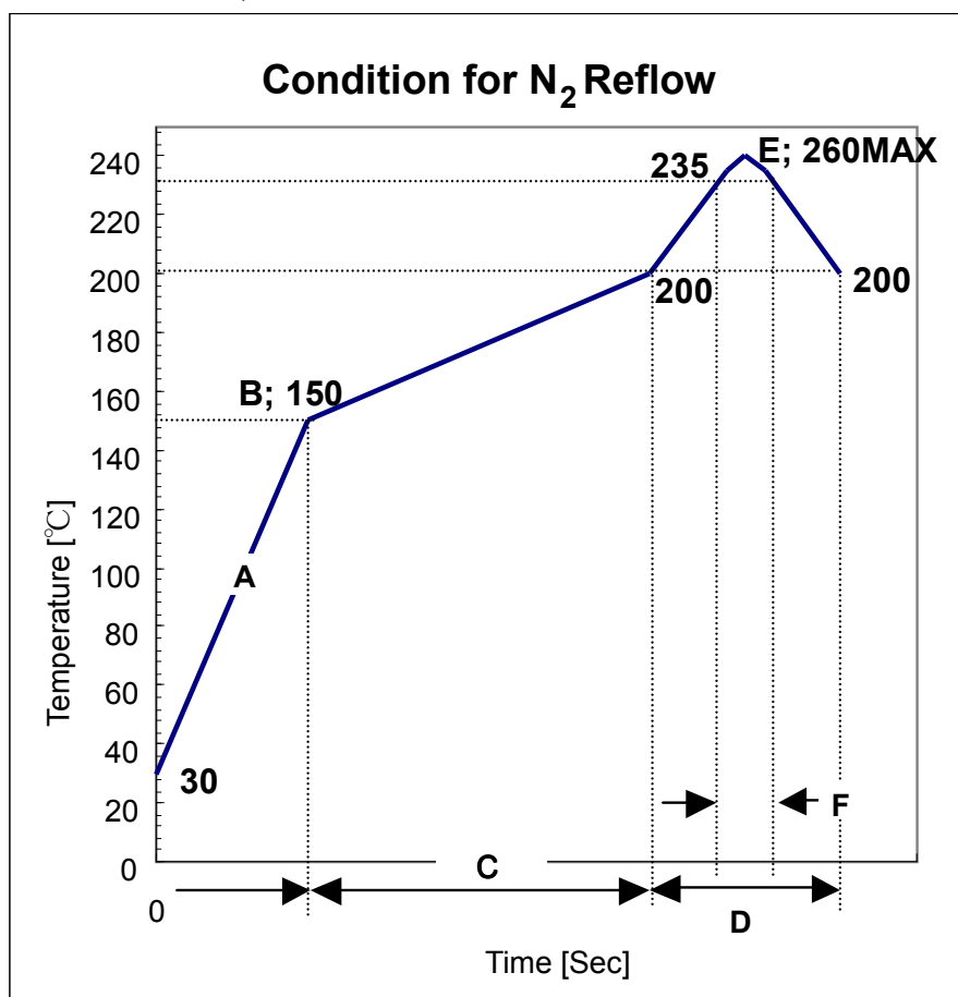
図 3 リフロープロファイル
