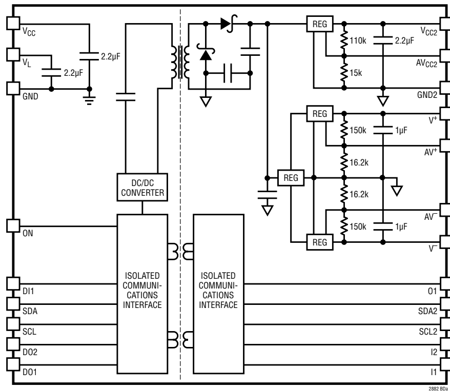
LTM2883-I
