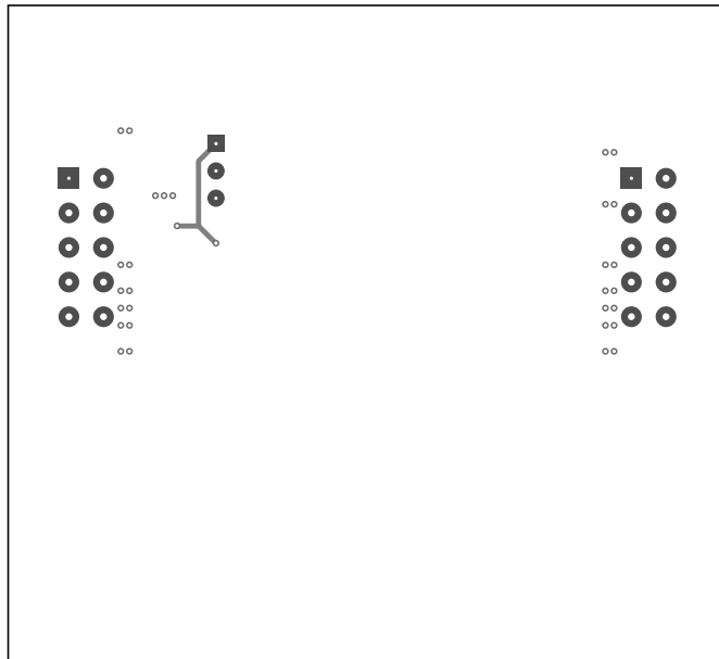
Inner Layer 2
