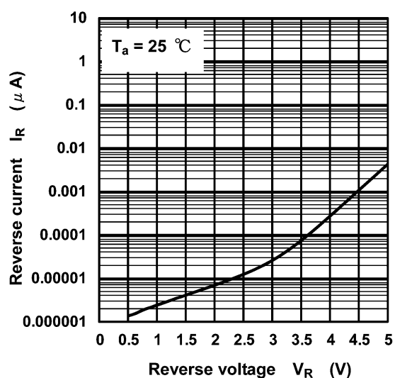
Fig. 8.2 I_R - V_R
