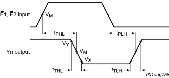
Fig. 7. Input ( \bar{E}1 , \bar{E}2 ) to output ( Yn ) propagation delays and output transition times
