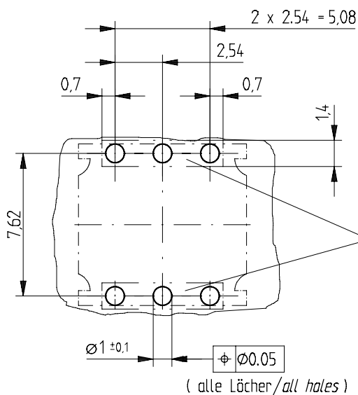
Leiterplattenbohrbild PCB drillhole pattern
