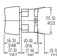
Extended Actuator
