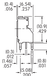
Extended Actuator
