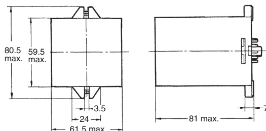
MM3P(N)
