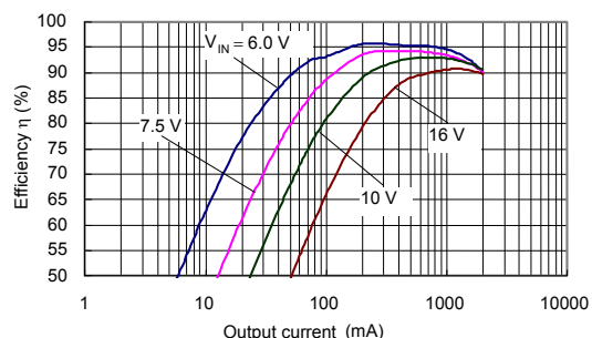
(23) S-8533A50AFT (CPH6302/CPH6402)
