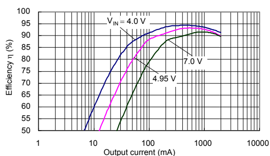
(21) S-8533A33AFT (CPH6302/CPH6402)
