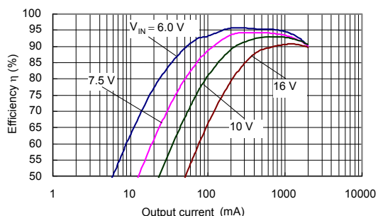
(23) S-8533A50AFT (CPH6302/CPH6402)
