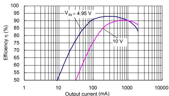
(23) S-8533A50AFT (CPH6302/CPH6402)
