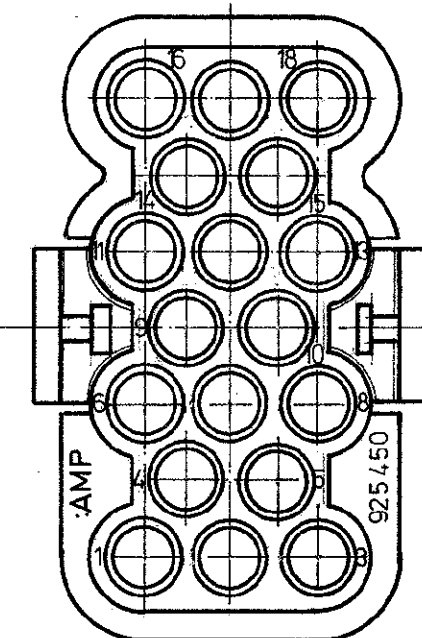
Ansicht "X"
