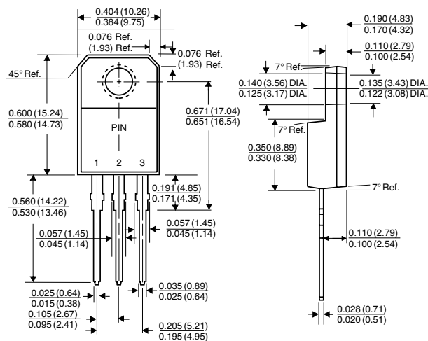
ITO-220AB
