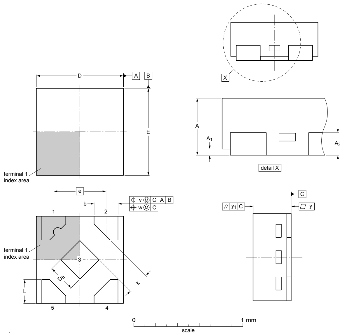
Dimensions
