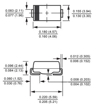
DO-214AA
