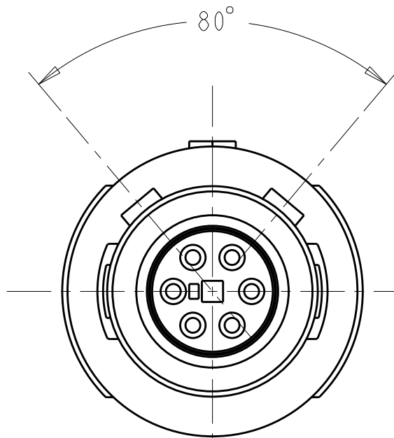
80° KEYING SCALE 4:1
