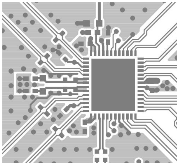
Top Side
