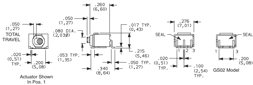
GS01MSABE Horizontal Actuation SPDT
