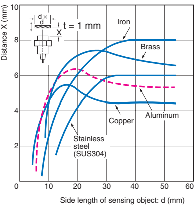
E2EZ-X8
