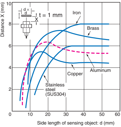
E2EZ-X8
