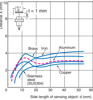
E2EZ-X4
